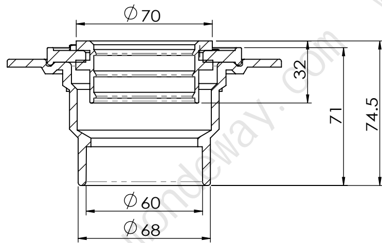
剖面 A-A
