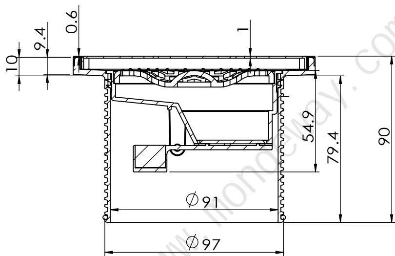
剖面 A-A
