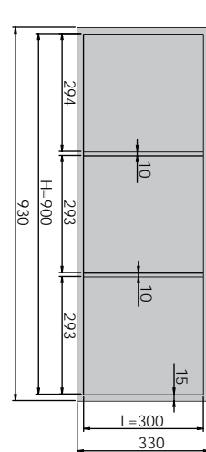
Model 30x90 cm
